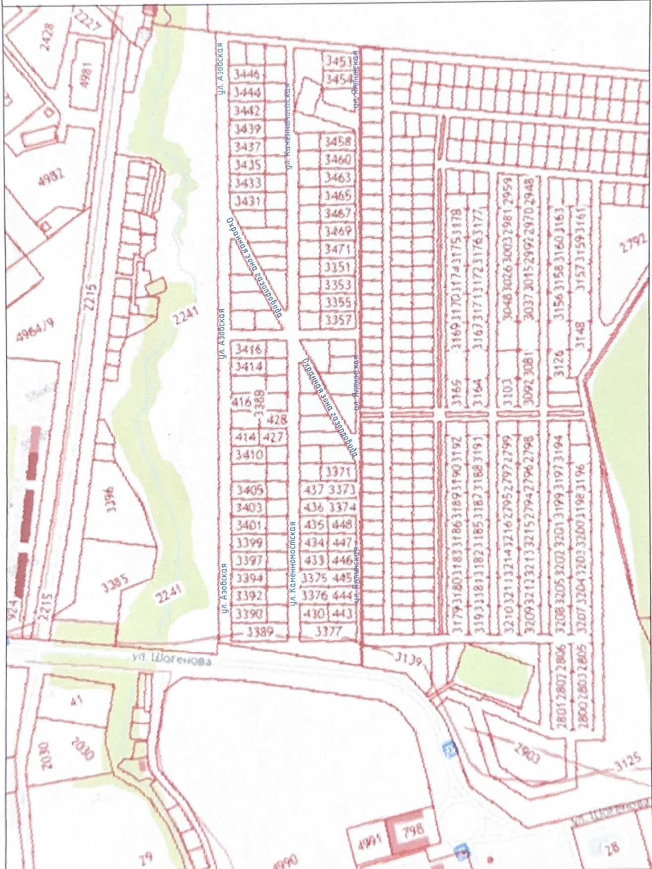
Схема расположения улично-дорожной сети мкр. Мишхидж (участок №2) г.о. Нальчик
